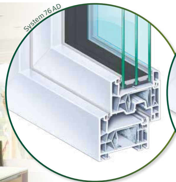
Profil 76 AD Profiltiefe 76mm Rahmen und Flügel mit Stahl verstärkt 5 Dämmkammern 2 Dichtungsebenen
